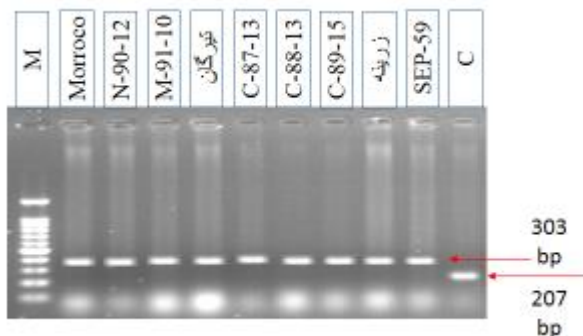
شکل ۳. شناسایی مکان ژنی Sr26 در ارقام و لاین‌های امیدبخش گندم بر روی ژل آگارز دو درصد به صورت نوار ۲۰۷ (حضور ژن) و ۳۰۳ (عدم حضور ژن) جفت بازی به ترتیب با استفاده از نشانگرهای اختصاصی Sr26#43 و BE518379 . از چپ به راست M: نشانگر وزنی DNA، رقم شاهد حساس به بیماری (Morocco)، لاین‌های منتخب گندم و C: رقم شاهد مثبت Eagle .
