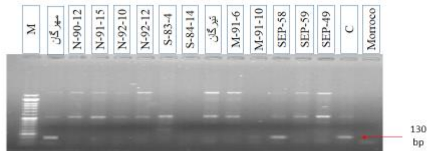
شکل ۲. شناسایی مکان ژنی Sr25/Lr19 در ارقام و لاین‌های امیدبخش گندم بر روی ژل آگاروز دو درصد به صورت نوار ۱۳۰ جفت بازی با استفاده از نشانگر اختصاصی Gb . از چپ به راست M: نشانگر وزنی DNA، لاین‌های منتخب گندم، C: رقم شاهد مثبت Agatha (CI 14048) / 9 * LMPG-6 DK1 (Morocco) و رقم شاهد حساس به بیماری (Morocco).
