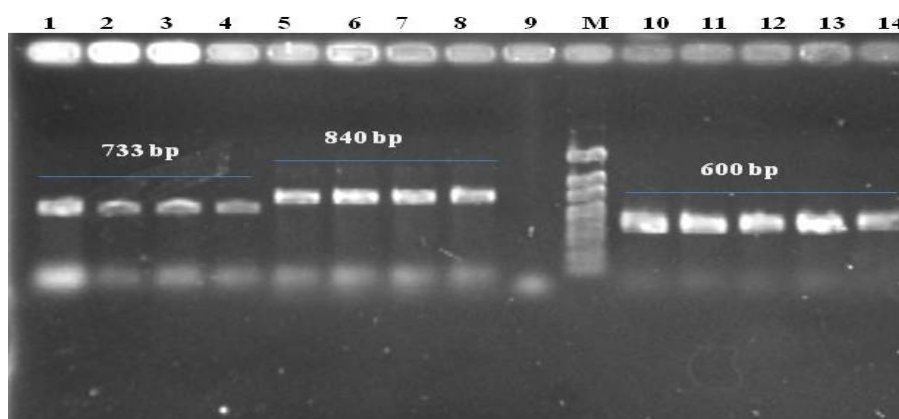
شکل ۳. نقوش الکتروفورزی محصول پی سی آر با استفاده از آغازگرهای اختصاصی Xylella fastidiosa . محصول PCR با جفت آغازگر RST31/RST33 از پرکنه‌های باکتری جداشده از مو (راهک های ۱ و ۲)، از نمونه دی ان ای دم برگ مو (راهک ۳)، از پرکنه‌های جدایه بادام (راهک ۴). محصول PCR با جفت آغازگر Dixon454fa/ Dixon1261rg از پرکنه باکتری جداشده از پسته (راهک ۵)، از نمونه دی ان ای دم برگ بادام (راهک ۶ و ۷)، از پرکنه‌های جدایه بادام (راهک ۸) و از پرکنه‌های جدایه مو (راهک ۹، تکثیر نشده). محصول PCR با جفت آغازگر 272-1-int/272-2-int از پرکنه‌های جدایه بادام (راهک ۱۰)، از نمونه دی ان ای دم برگ پسته (راهک ۱۱)، و از پرکنه‌های جدایه مو (راهک ۱۲ و ۱۳) و از نمونه دی ان ای دم برگ مو (راهک ۱۴). مارکر دی ان ای 100 bp (راهک M).
