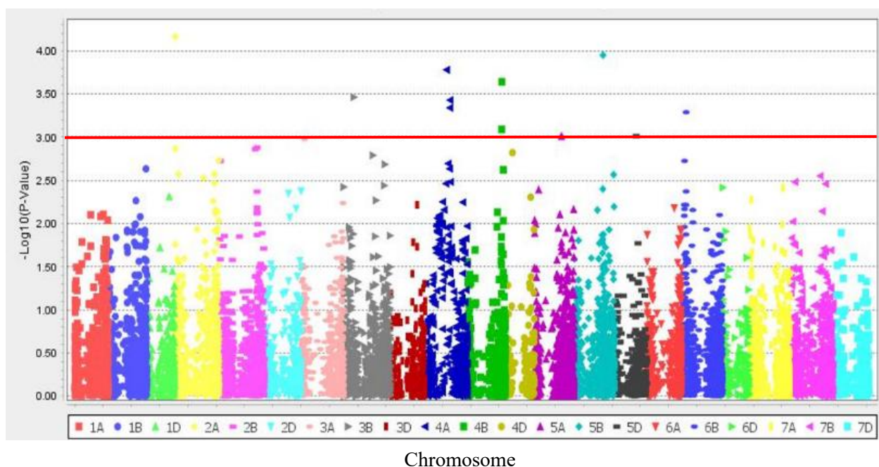
شکل ۳. پلات منهتن، نشان‌دهنده نواحی ژنومی مرتبط با مقاومت به Heterodera filipjevi در ژنوتیپ‌های گندم، بر اساس مدل خطی عمومی (GLM). محور افقی (X) موقعیت نشانگرهای SNP را روی کروموزوم‌های گندم و محور عمودی (Y) مقادیر -\log_{10}(p\text{-value}) به ارتباط نشانگر-صفت نشان می‌دهد. خط قرمز، آستانه معنی‌داری در سطح کل ژنوم را نشان می‌دهد.
