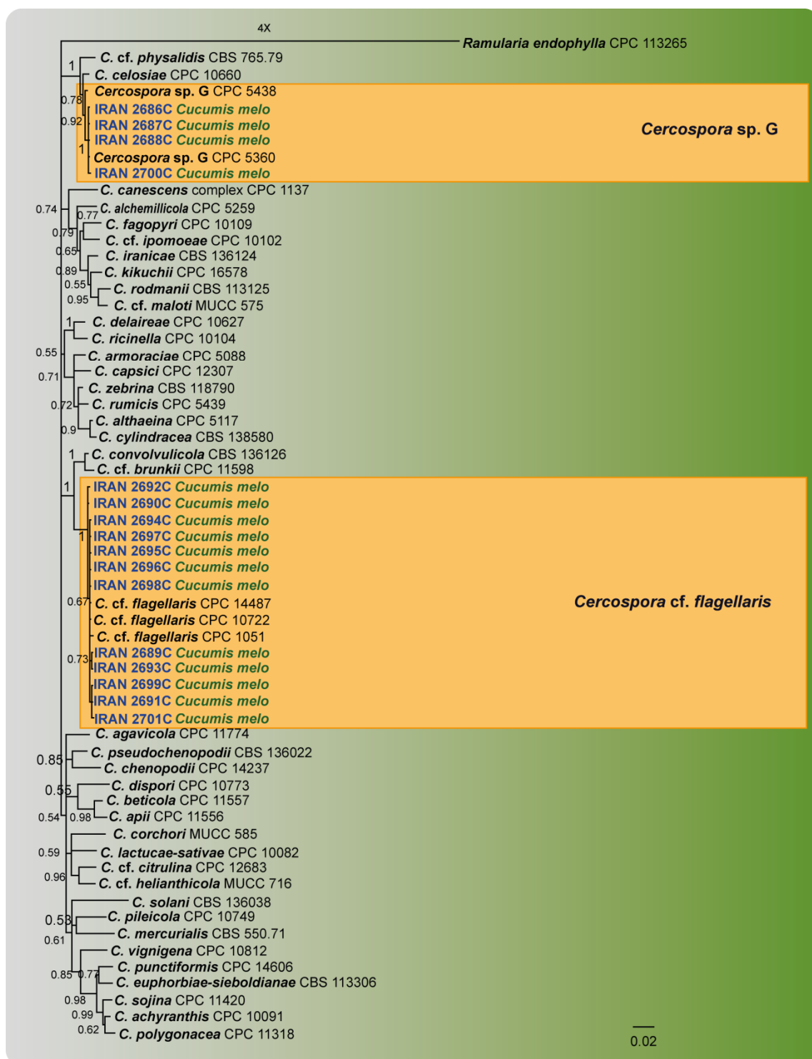
شکل ۲. تبارنمای فیلوژنتیکی حاصل از استنتاج بیژیان با استفاده از ترکیب توالی پنج ناحیه ژنی ITS، actA ، tef1 ، cmdA و his3 جدایه-های سرکوسپورای بدست‌آمده از گیاه خربزه در استان گیلان. این تبارنما نسبت به گونه Ramularia endophylla (جدایه CPC 113265) ریشه‌یابی شده است.
